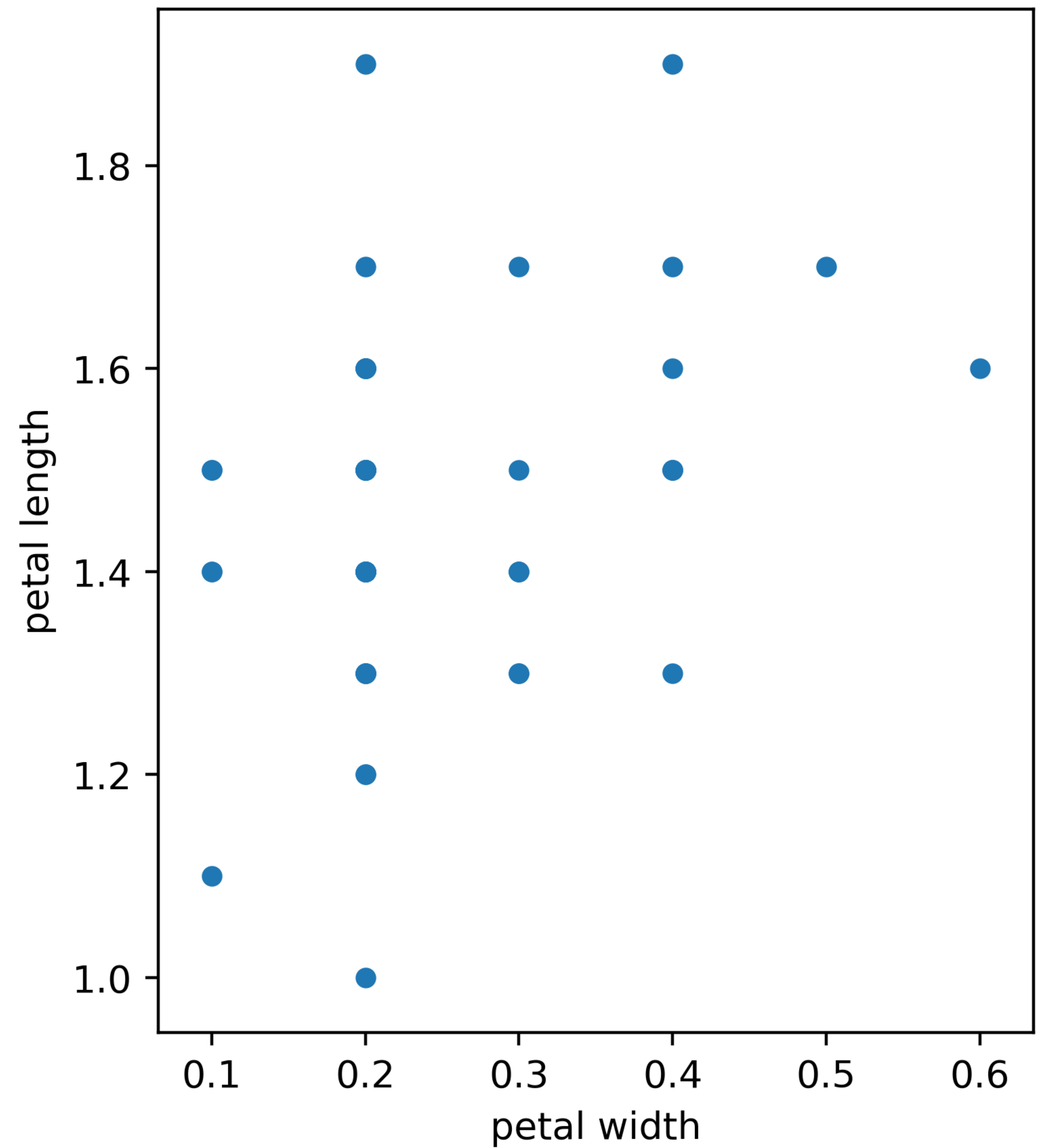
setosa
