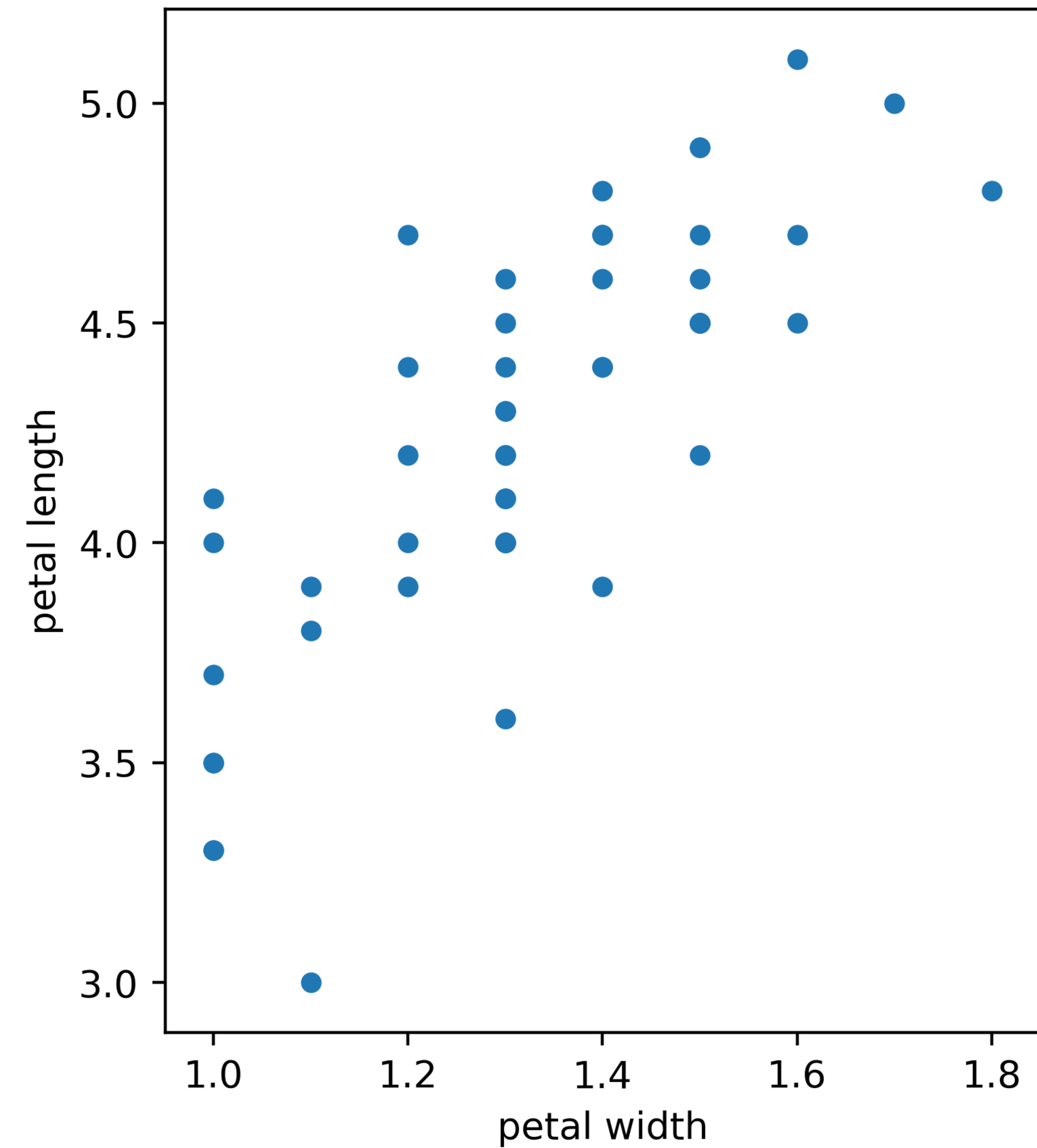
versicolor
