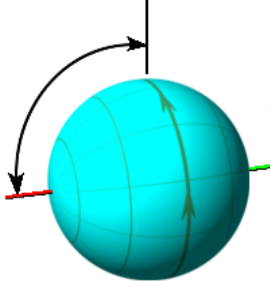
Uranus: 97^\circ
