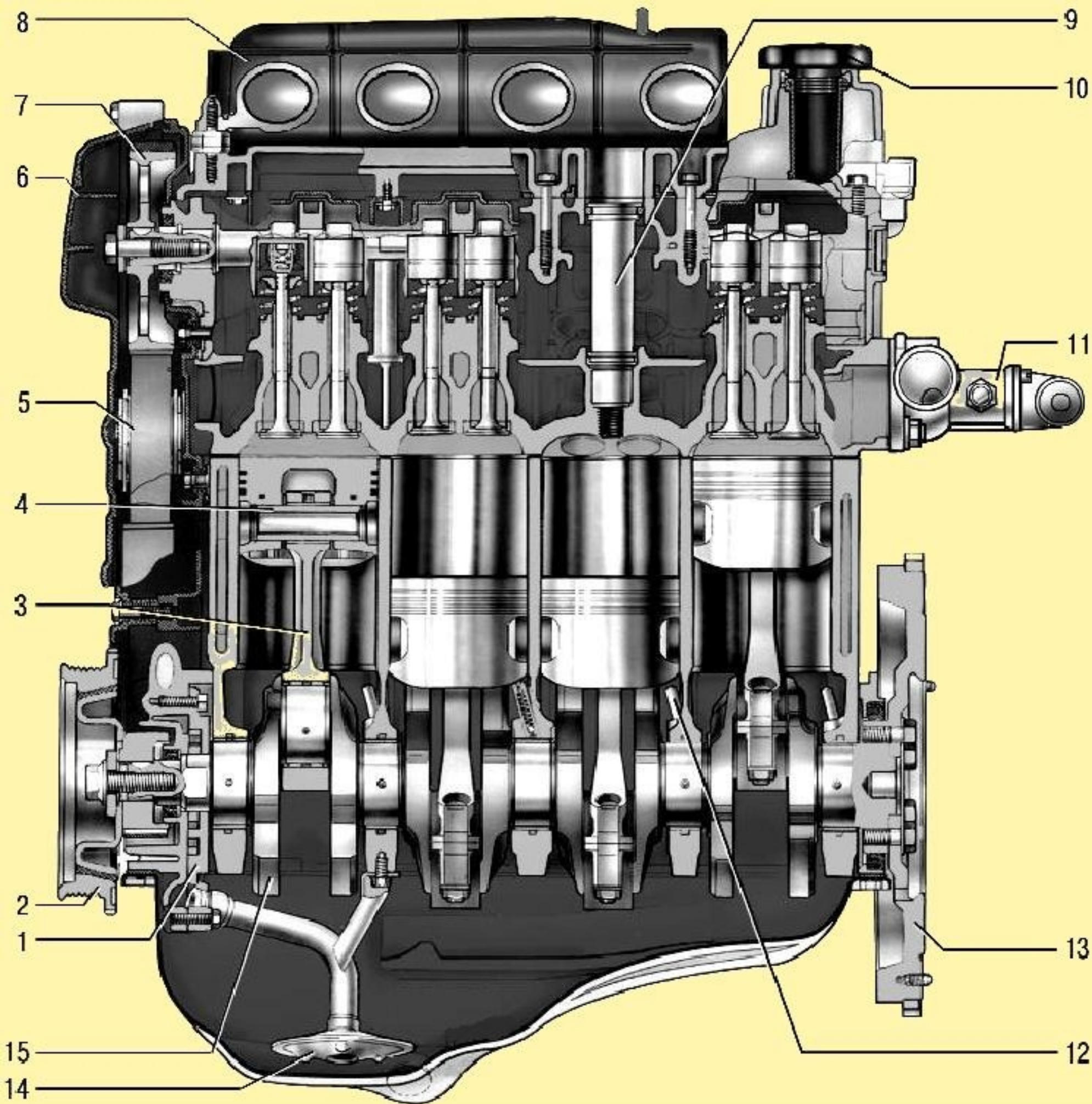
Продольный разрез двигателя ВАЗ-21126: 1 – масляный насос; 2 – шкив привода генератора; 3 – шатун; 4 – поршневой палец; 5 – ремень привода газораспределительного механизма; 6 – крышка газораспределительного механизма; 7 – шкив распределительного вала; 8 – впускной коллектор; 9 – свечной колодец; 10 – крышка маслосливной горловины; 11 – термостат; 12 – маховик; 13 – форсунка охлаждения дна поршня; 14 – маслоприемник; 15 – коленчатый вал
