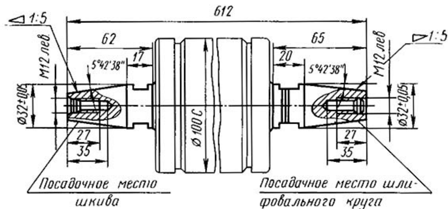
Эскиз концов шлифовальной головки
