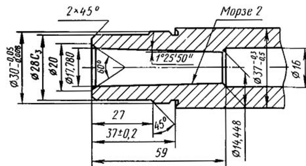
Эскиз конца шпинделя прибора праки
