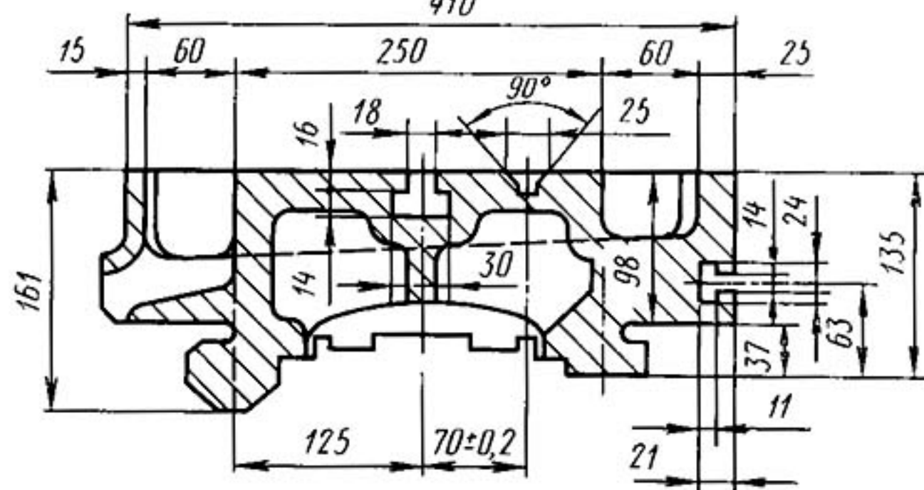
Эскиз стола
