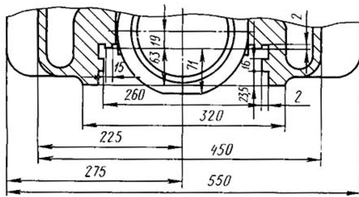
Эскиз направляющей колонки
