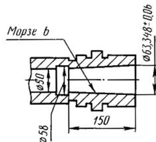
Эскиз переднего конца шпинделя механизма деления
