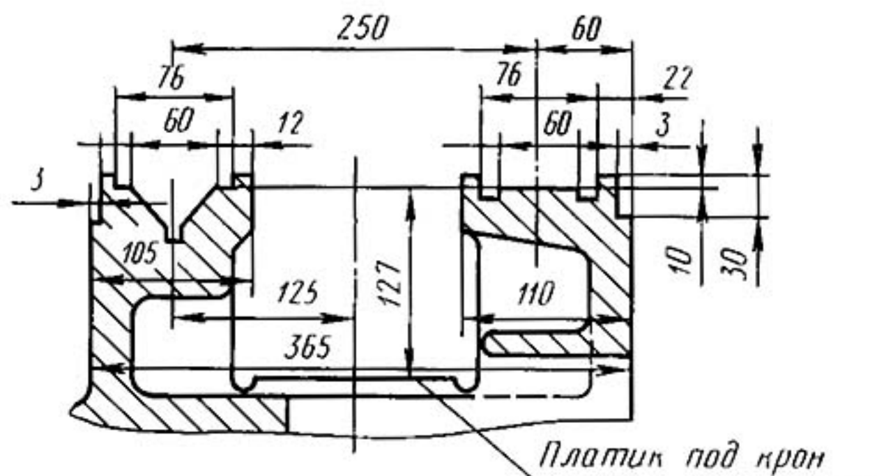
Эскиз направляющей станины
