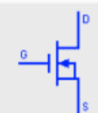
Enhancement Type MOSFET
