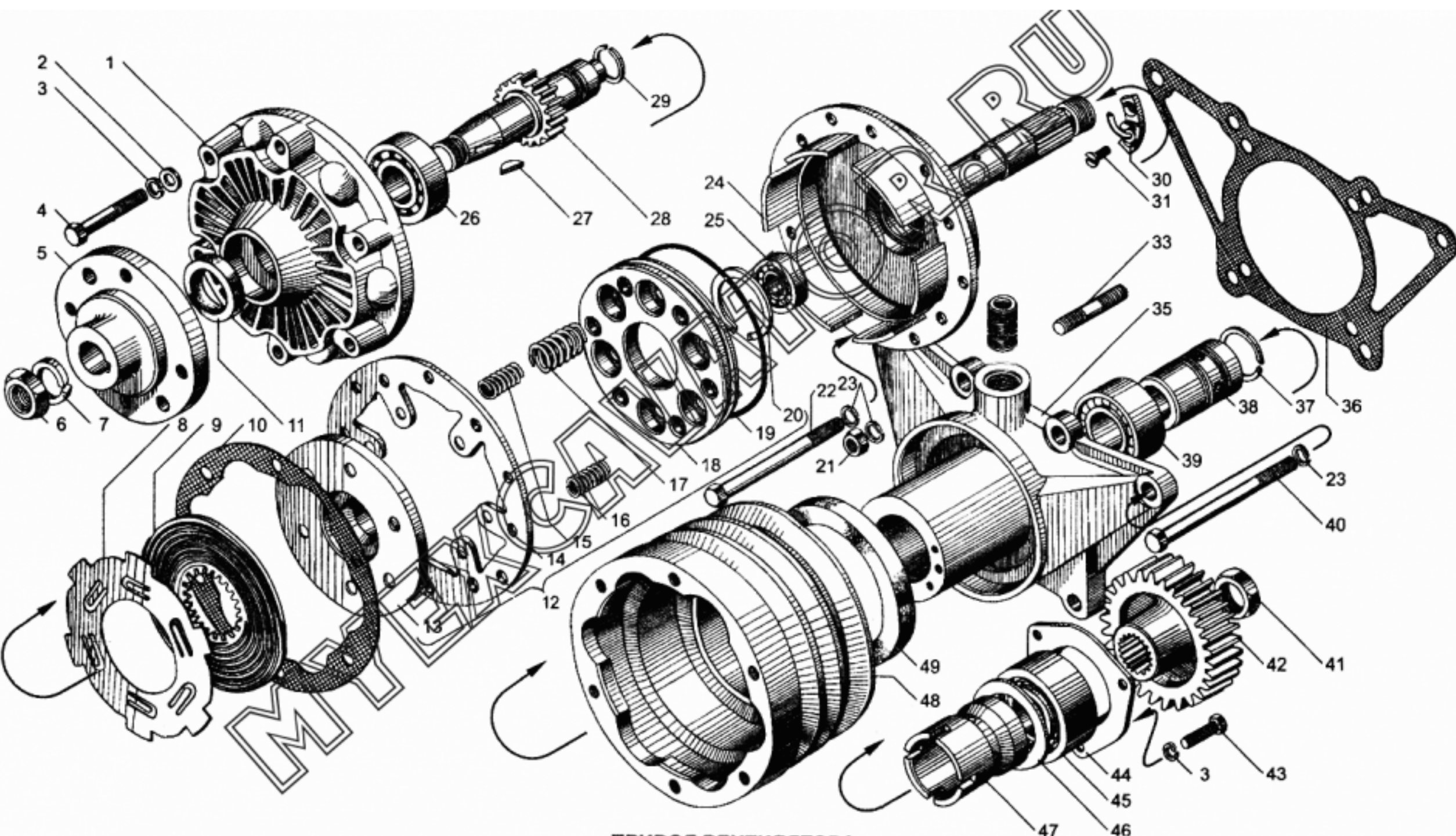
ПРИВОД ВЕНТИЛЯТОРА
