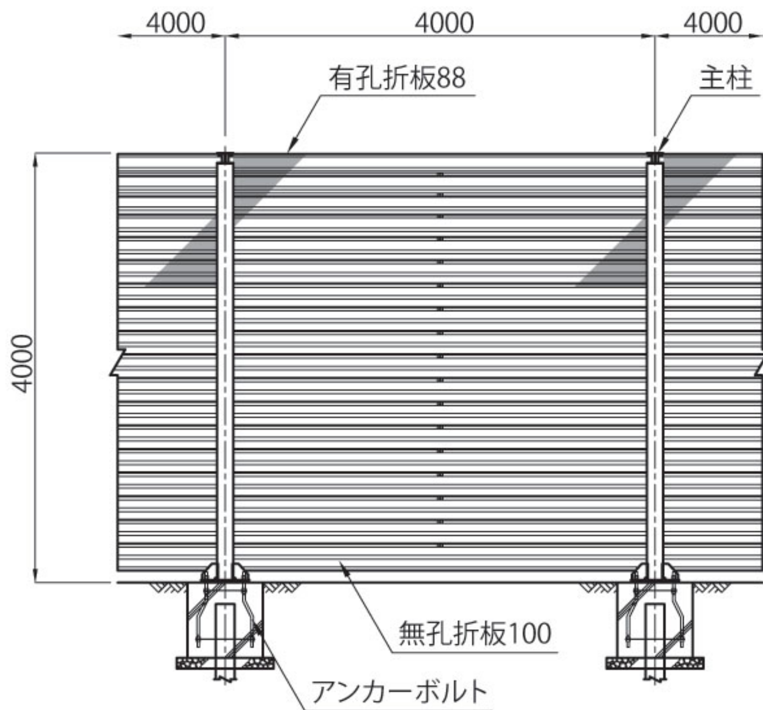
立面図
