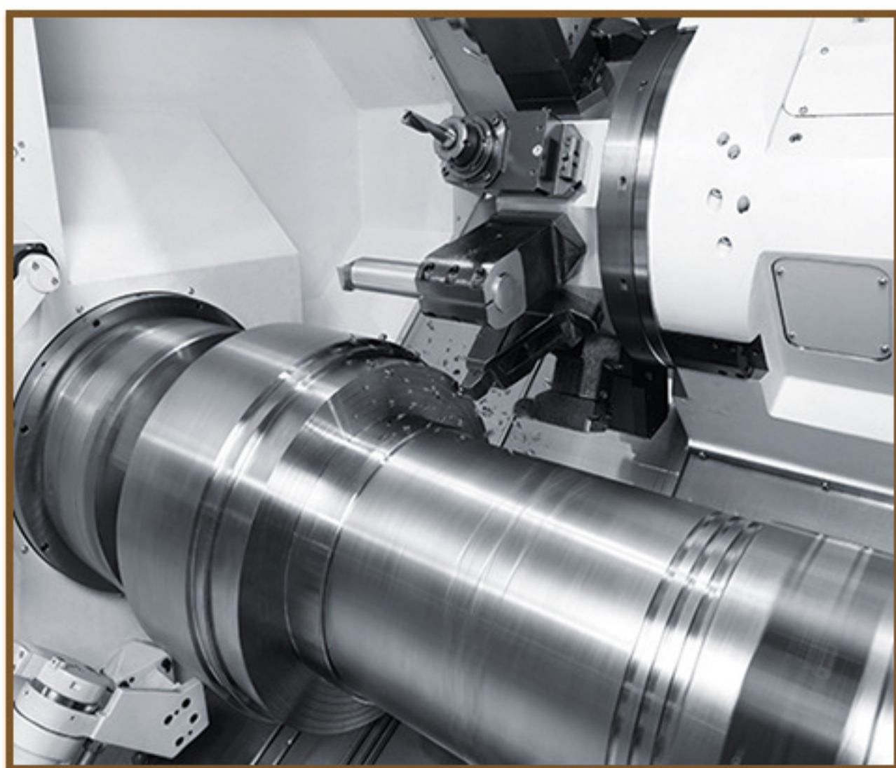
车削加工
