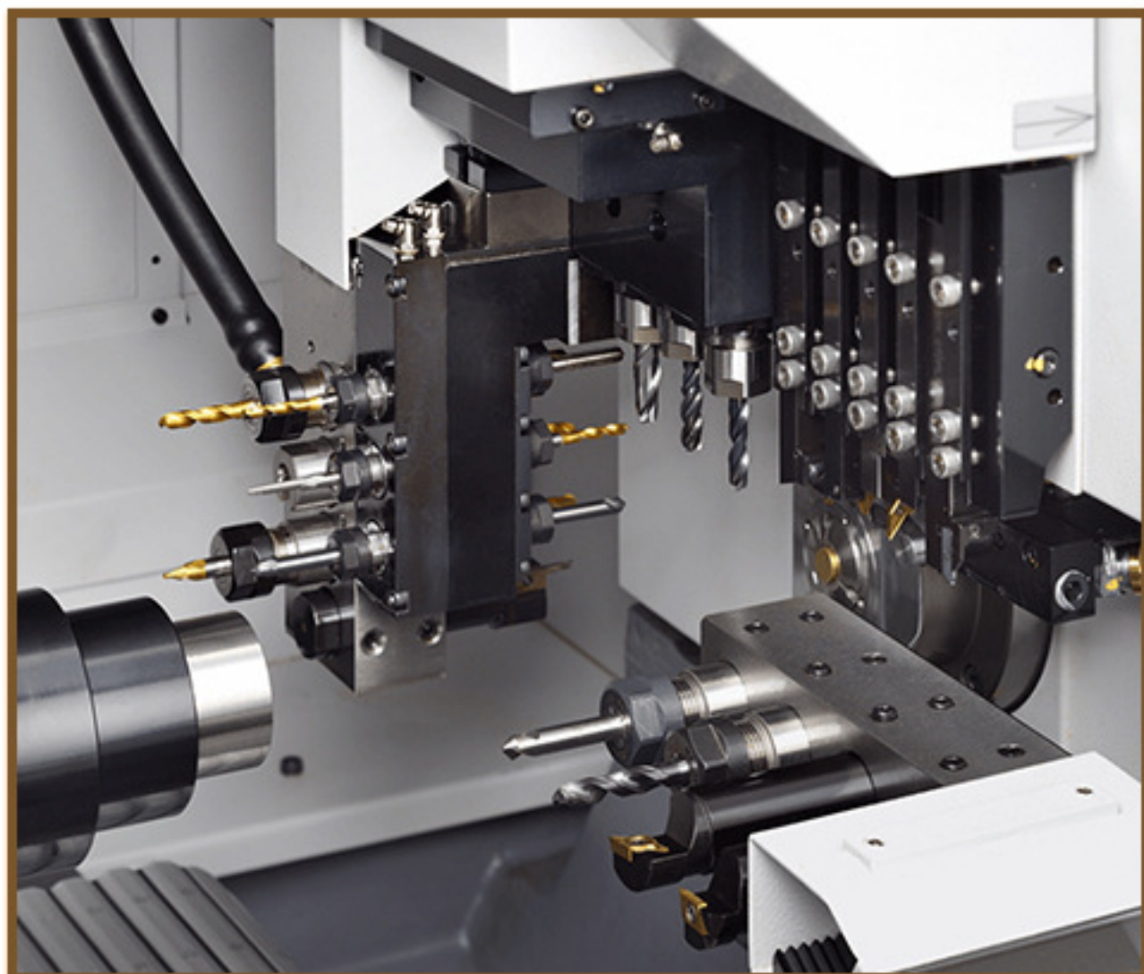
走心机加工
